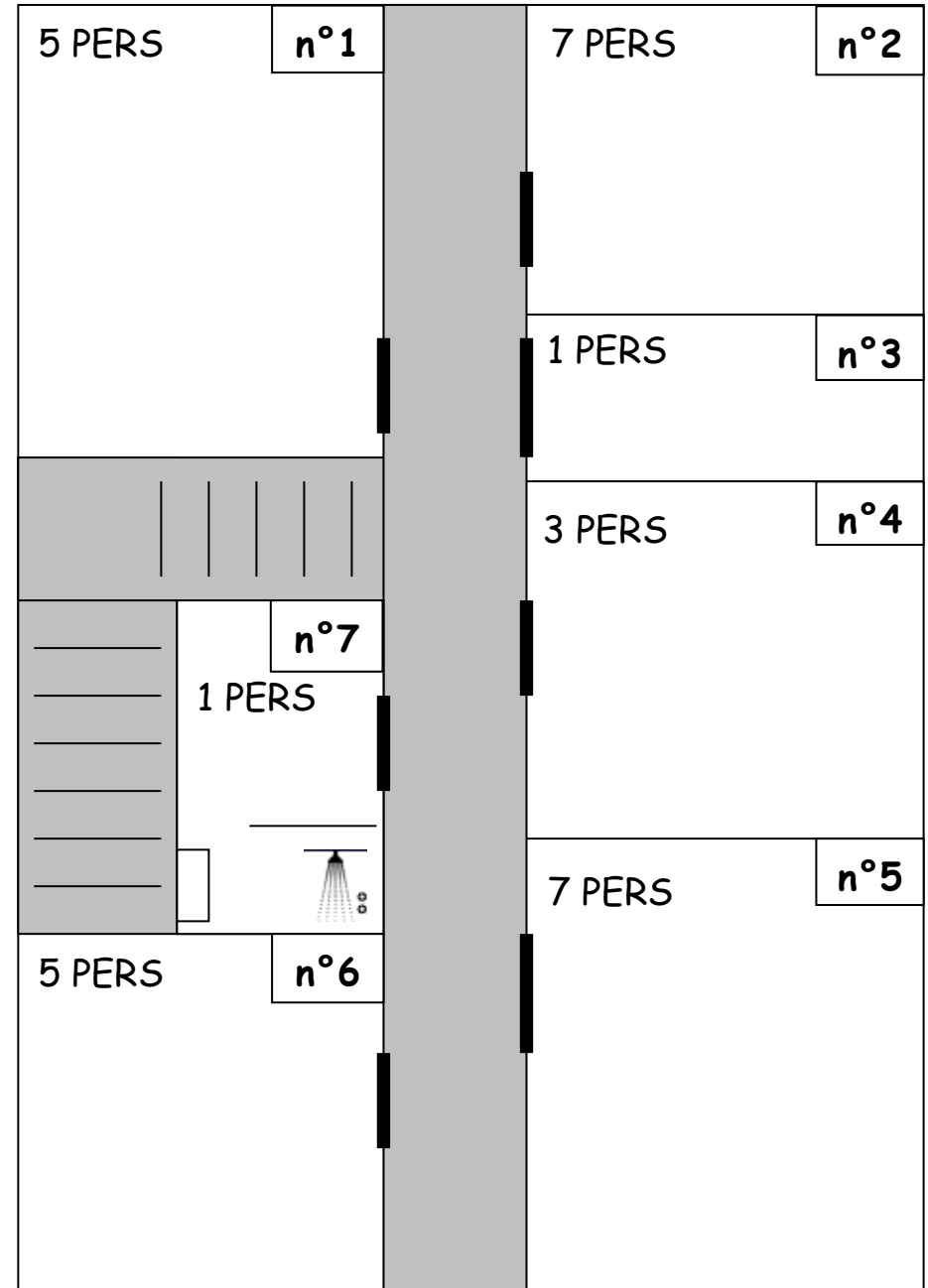
1° Obergeschoss - Etage-Verdieping
